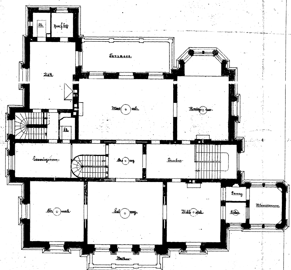
Grundplan af 1 sta vån.
