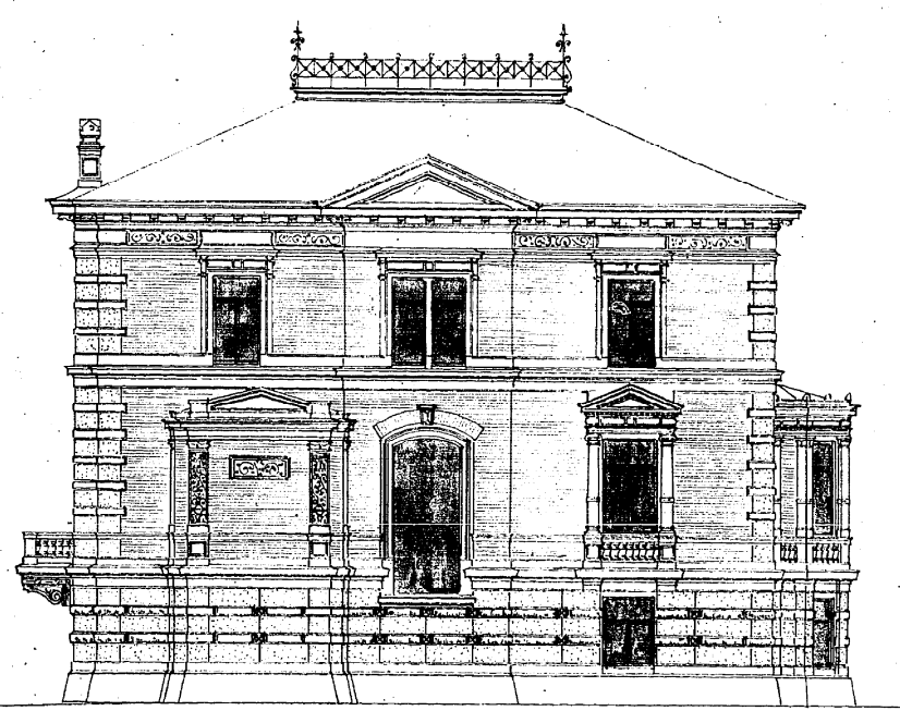
Fasade åt Vasier.
