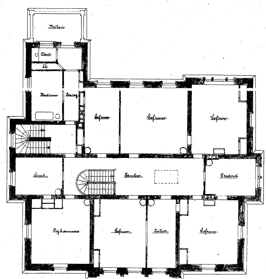
Grundplan af 2 da vån.
