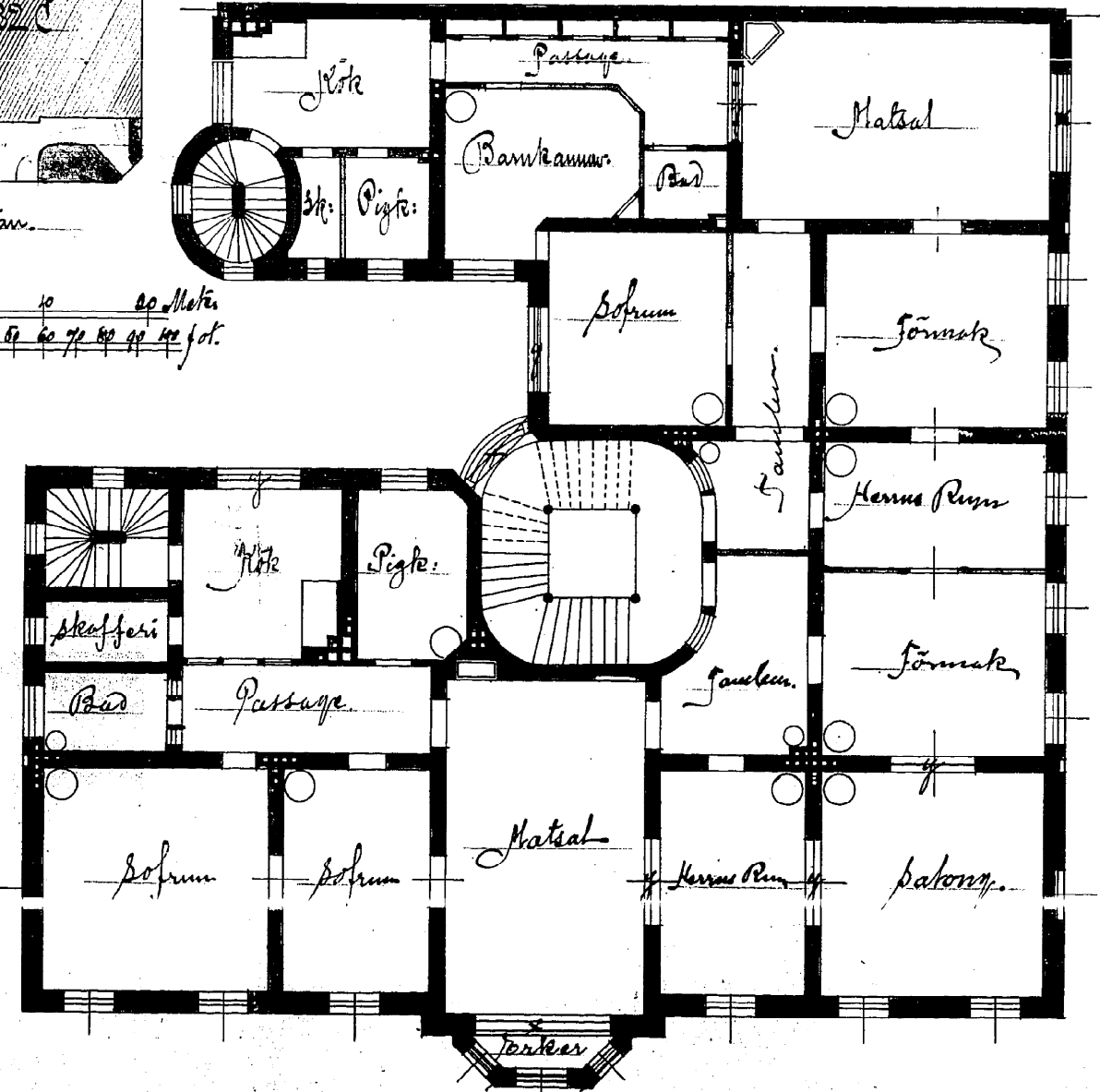
Plan af 3 de Våning
