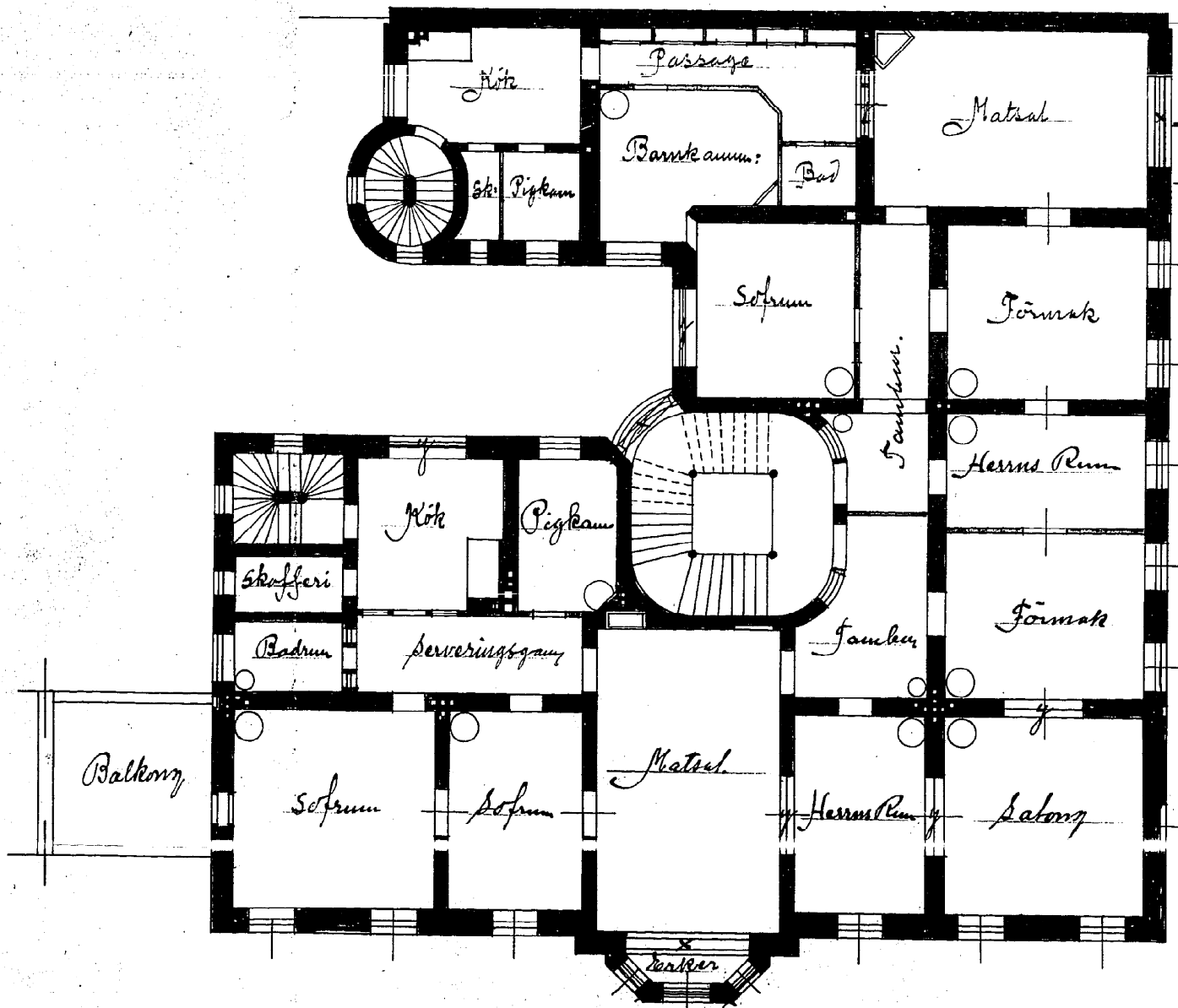
Plan af 2 da Våning
