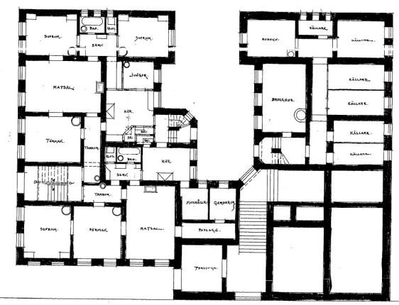
PLAN AF BOTTENVÄK
