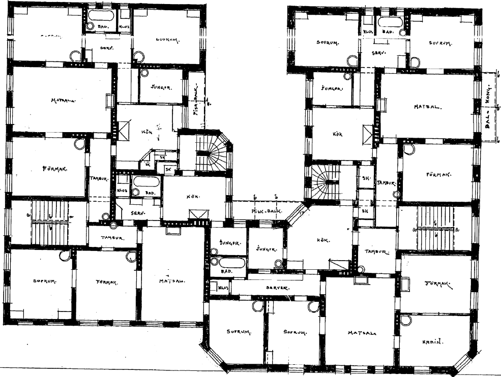
PLAN AF VÅN 4TR. UPP.
