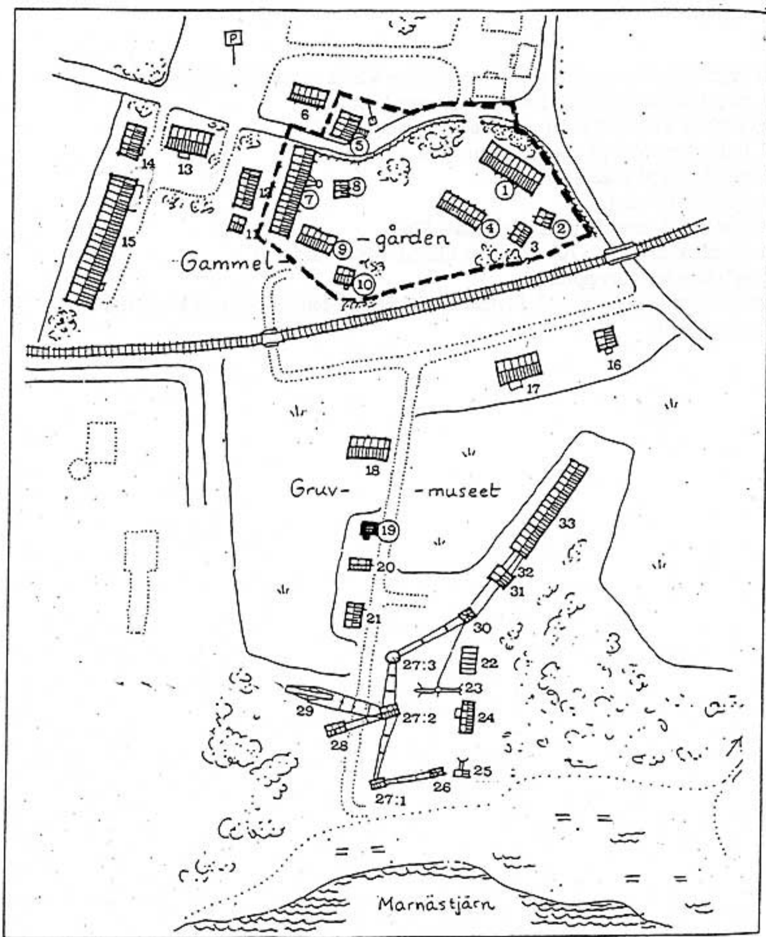
SITUATIONSPLAN BERGSMANSGÅRDEN PÅ LUDVIKA GAMMELGÅRD
