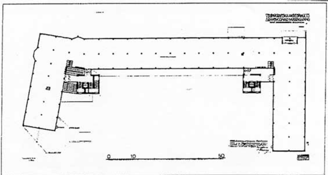
Lithografen, huvudbyggnad och flyglar (A). Utdrag ur L. Brunnström, Den rationella fabriken
