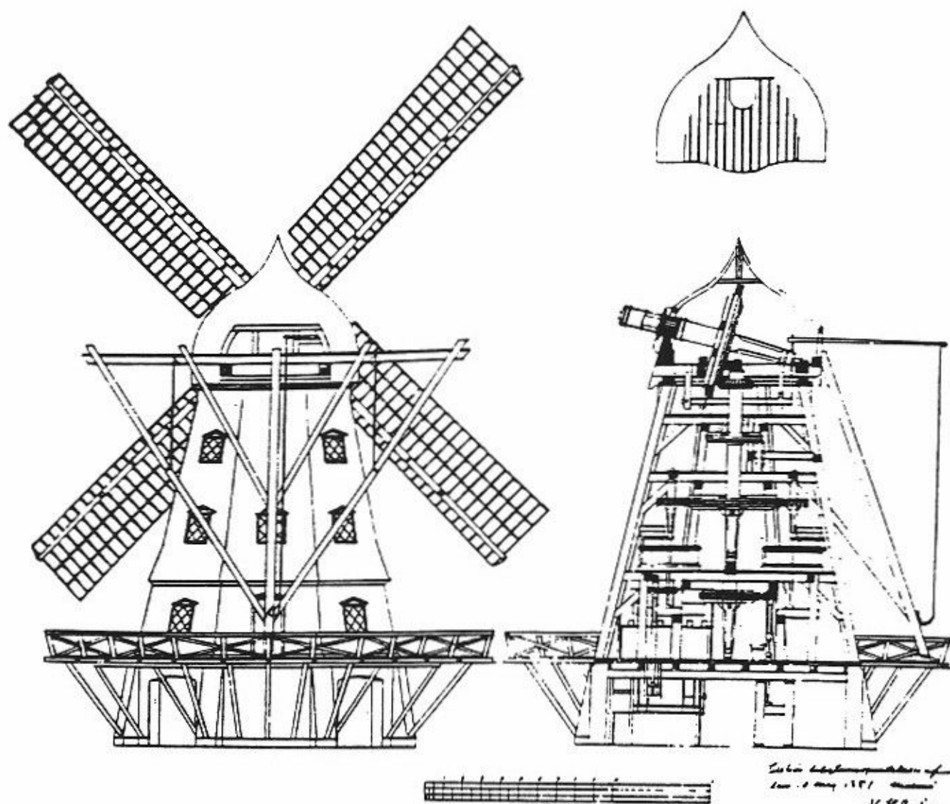
Byggnadsritning av Slottsmöllan godkänd 1851. Original i Krigsarkivet i Stockholm.
