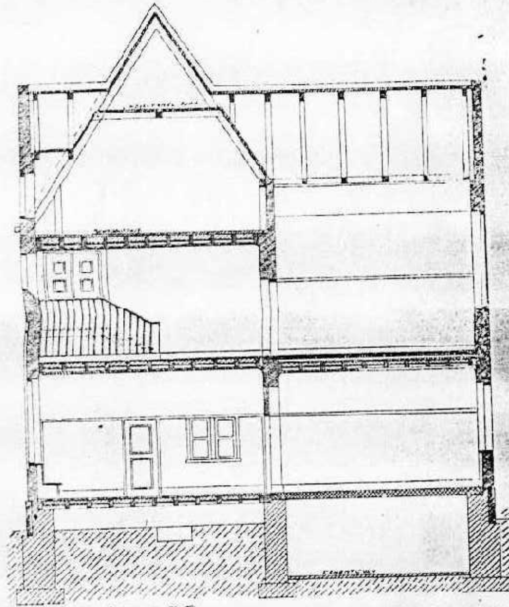
SEKTION D-D
