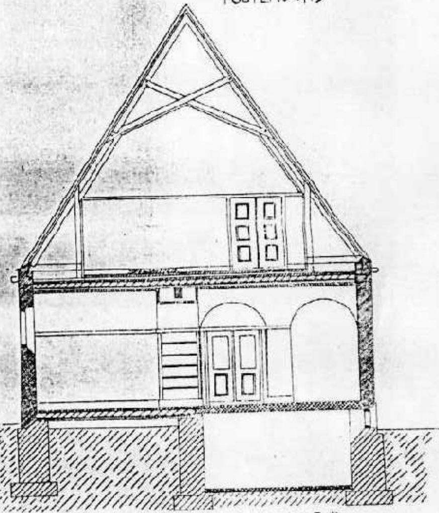
SEKTION A-A
